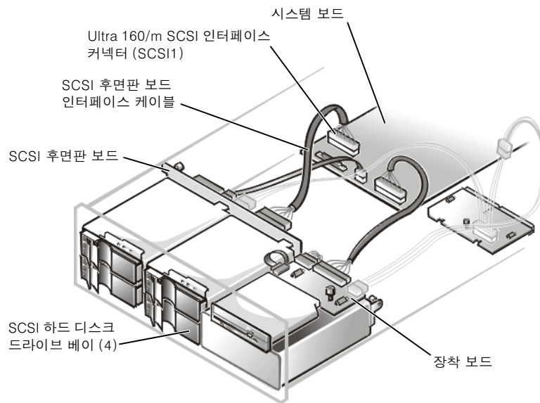
그림 7-1. 하드 디스크 드라이브 하드웨어
