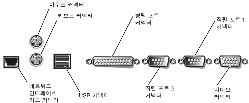
그림 B-1. I/O 포트 및 커넥터
