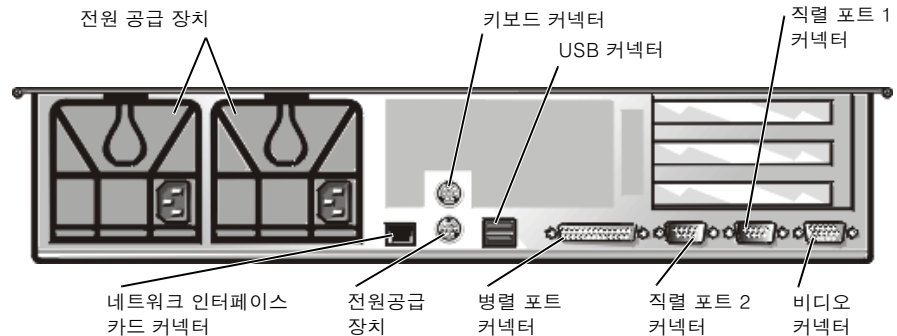
그림 1-2. 후면 패널 구조
