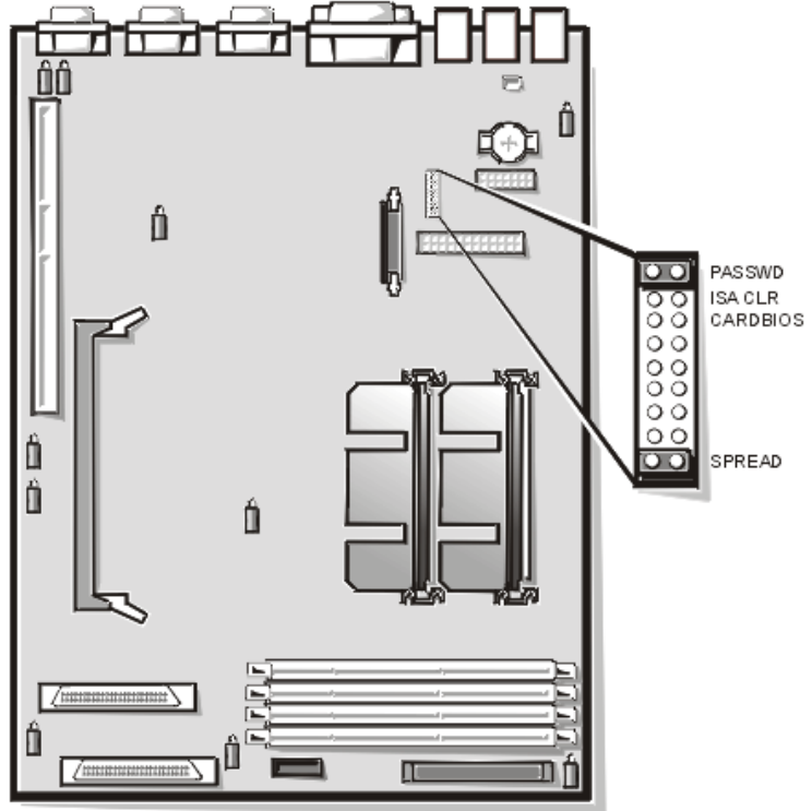
그림 6-3. 시스템 보드 점퍼
