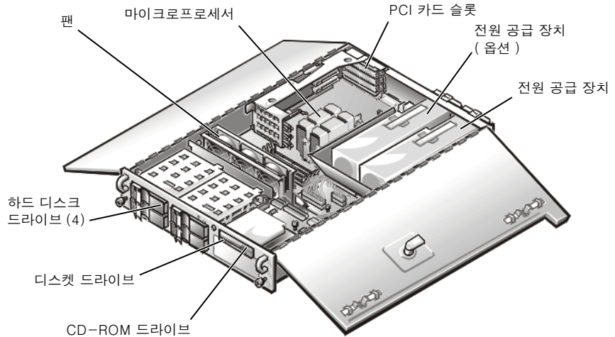
그림 6-2. 시스템 내부 ( 위에서 본 모습 )
