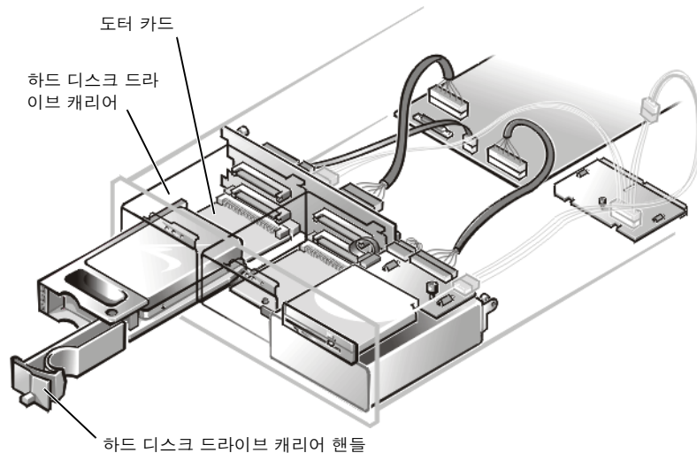
그림 7-2. SCSI 하드 디스크 드라이브 캐리어 설치
